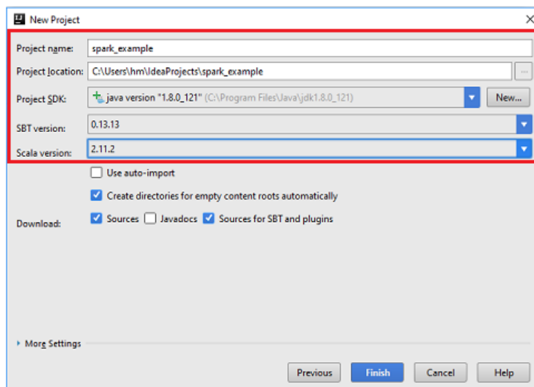
Εικόνα 8 - Project Configurations
