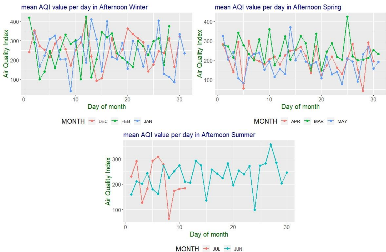
Γράφημα 25: Γραφήματα μέσω των τιμών AQI τις μεσημεριανές ώρες ανά εποχή.
