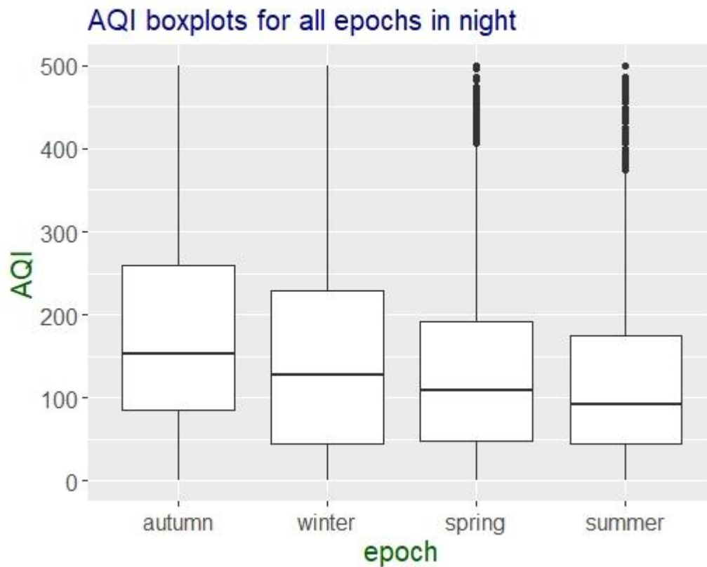
Γράφημα 22: Boxplots φαίνεται η κατανομή των τιμών AQI τις βραδινές ώρες ανά εποχή
