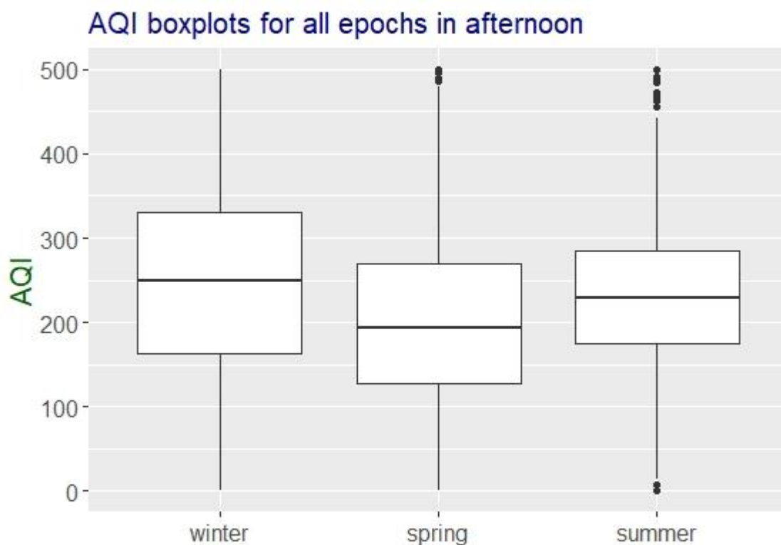
Γράφημα 26: Boxplots φαίνεται η κατανομή των τιμών AQI τις μεσημεριανές ώρες ανά εποχή
