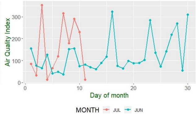
Γράφημα 17: Γραφήματα μέσω των τιμών AQI τις μεσημεριανές ώρες ανά εποχή.
