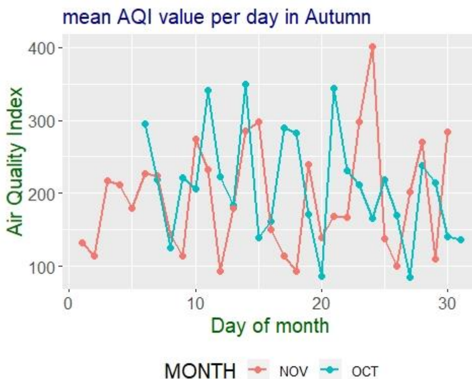
Γράφημα 8: Μέσες τιμές των εγγραφών AQI ανά ημέρα για τον αισθητήρα 8200015E την εποχή του φθινοπώρου.
