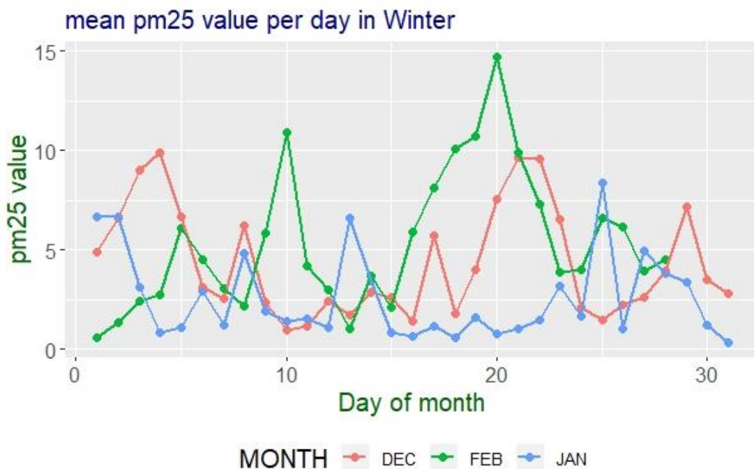
Γράφημα 2: Μέσες τιμές ανά ημέρα για τον αισθητήρα 8200015E την εποχή του χειμώνα
