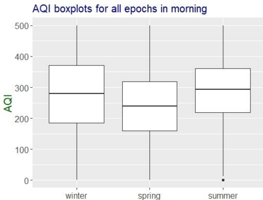
Γράφημα 24: Boxplots φαίνεται η κατανομή των τιμών AQI τις πρωινές ώρες ανά εποχή
