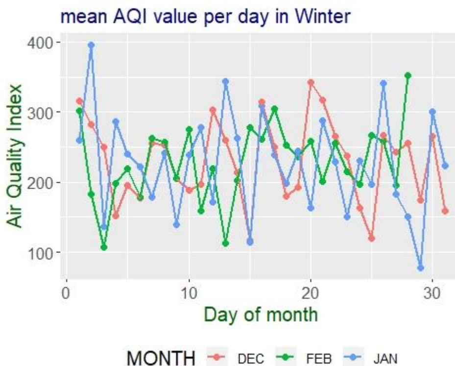
Γράφημα 12: Μέσες τιμές των εγγραφών AQI ανά ημέρα για τον αισθητήρα 8200015F την εποχή του χειμώνα.
