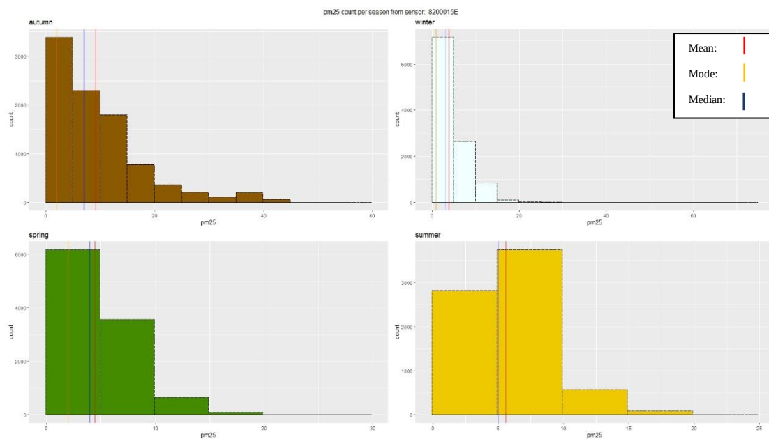
Εικόνα 5: Ιστόγραμμα που δείχνει το σύνολο των τιμών ανά εποχή για τον αισθητήρα 8200015E
