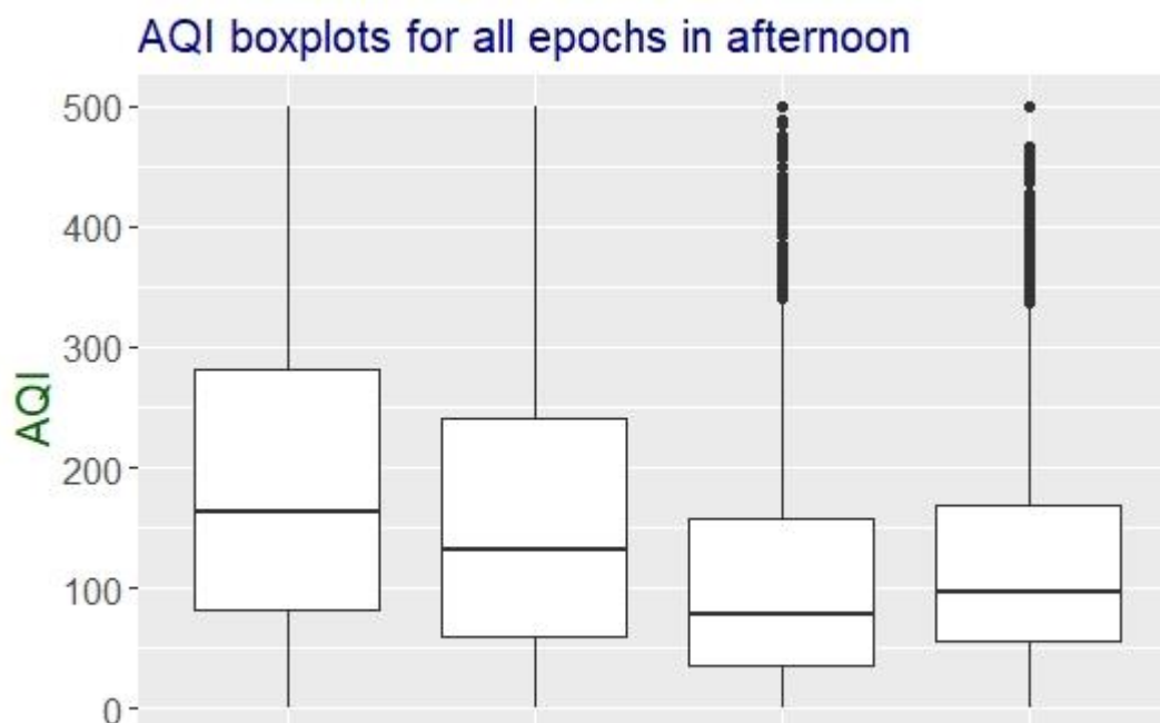
Γράφημα 18: Boxplots φαίνεται η κατανομή των τιμών AQI τις μεσημεριανές ώρες ανά εποχή
