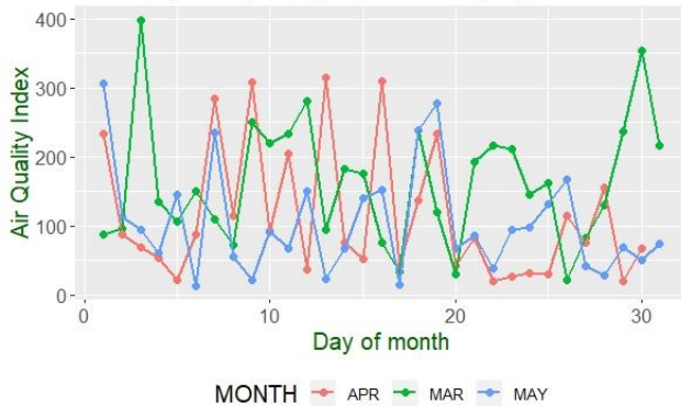
Γράφημα 17: Γραφήματα μέσω των τιμών AQI τις μεσημεριανές ώρες ανά εποχή.
