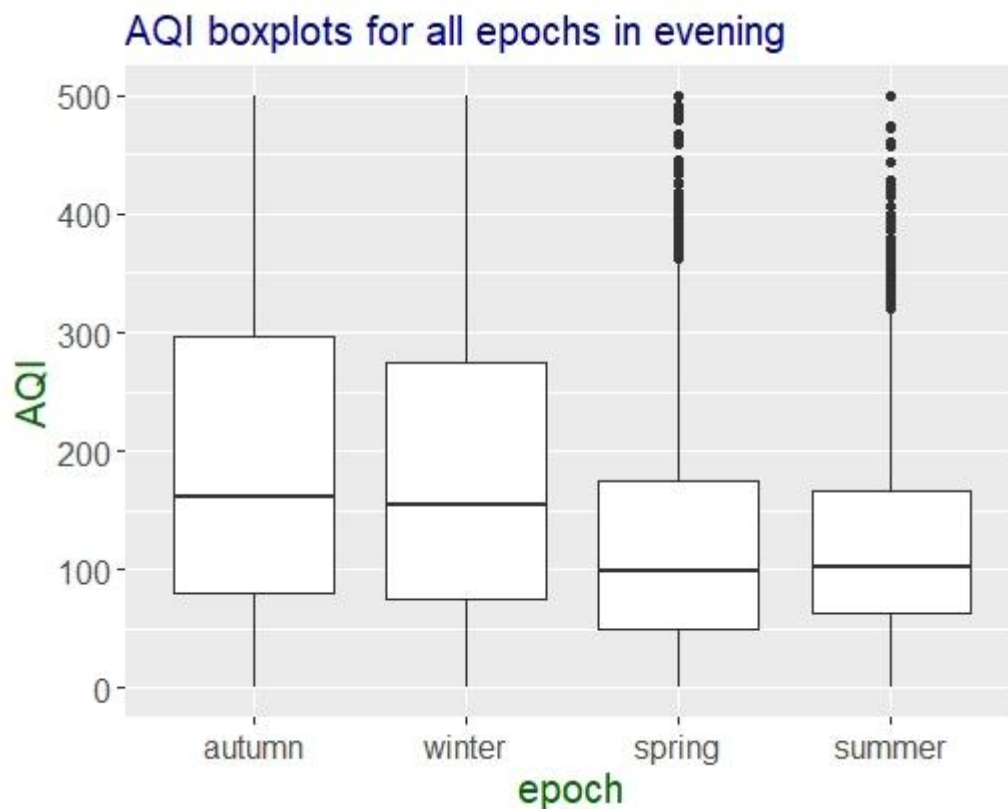
Γράφημα 20: Boxplots φαίνεται η κατανομή των τιμών AQI τις απογευματινές ώρες ανά εποχή
