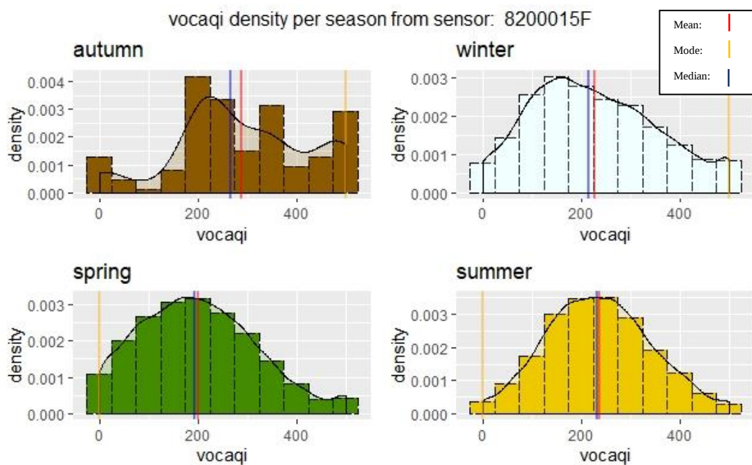
Εικόνα 10: Ιστογράμματα δημιουργημένα ανά εποχή για την τα σωματίδια AQI για τον αισθητήρα 8200015F. Στον κάθετο άξονα βλέπουμε την πιθανότητα της ύπαρξης των τιμών.
