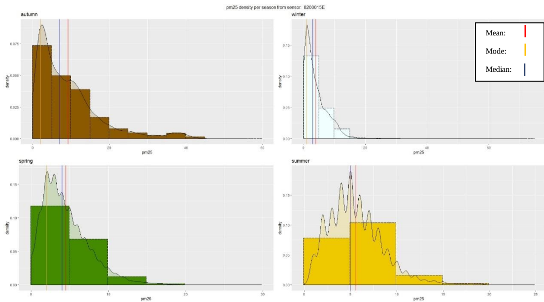
Εικόνα 4: Ιστογράμματα δημιουργημένα ανά εποχή για την τα σωματίδια pm_{25} για τον αισθητήρα 8200015E. Στον κάθετο άξονα βλέπουμε την πιθανότητα της ύπαρξης των τιμών. Ικανοποιητικές τιμές για την μέτρηση των σωματιδίων είναι τα 50\mu g/m^3 κατά μέσο όρο σε 24 ώρες.
