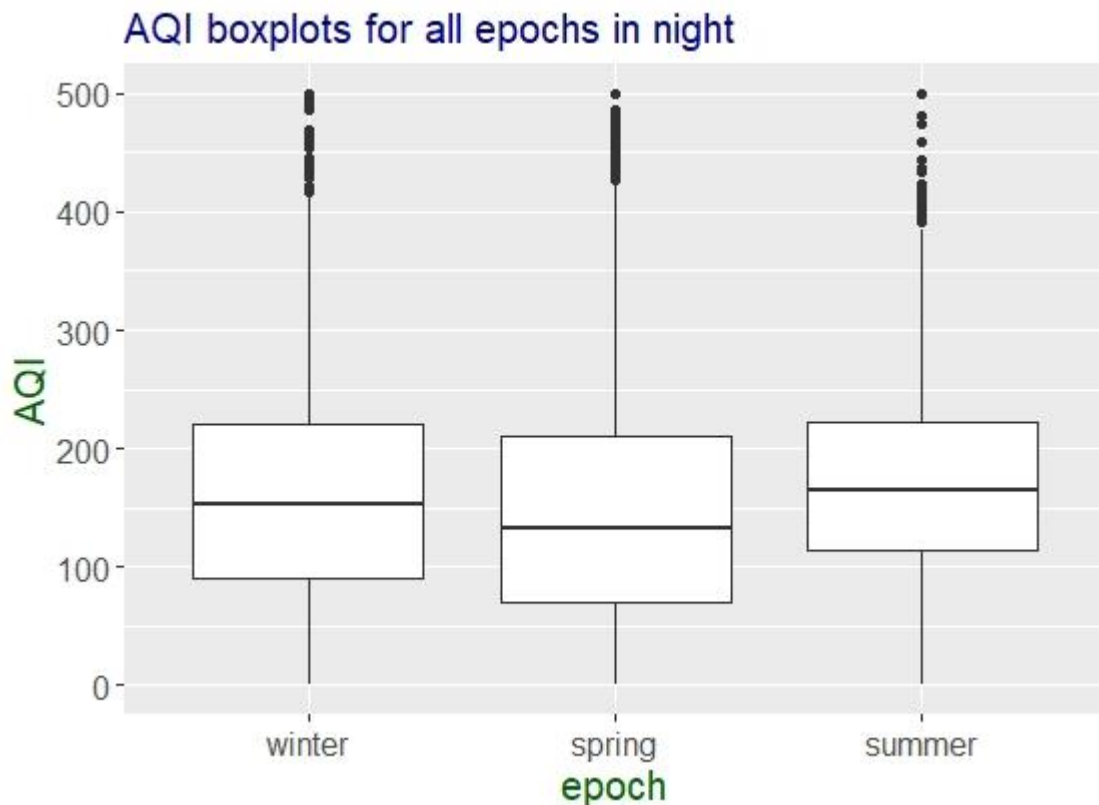
Γράφημα 30: Boxplots φαίνεται η κατανομή των τιμών AQI τις βραδινές ώρες ανά εποχή.
