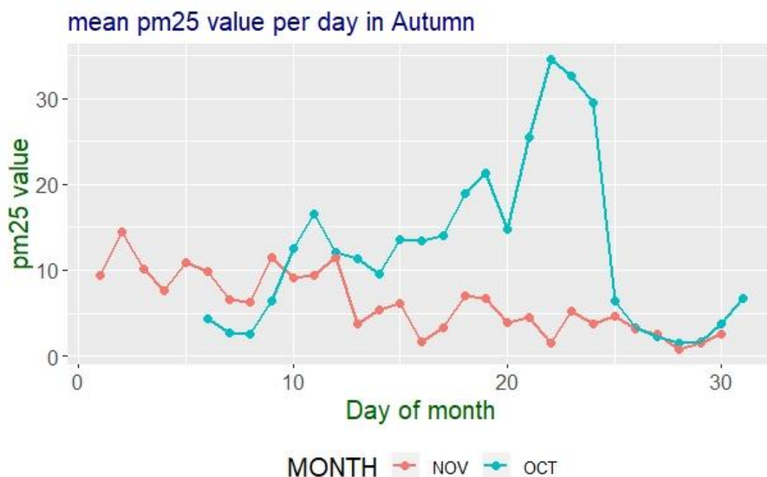
Γράφημα 1: Μέσες τιμές ανά ημέρα για τον αισθητήρα 8200015E την εποχή του φθινοπώρου
