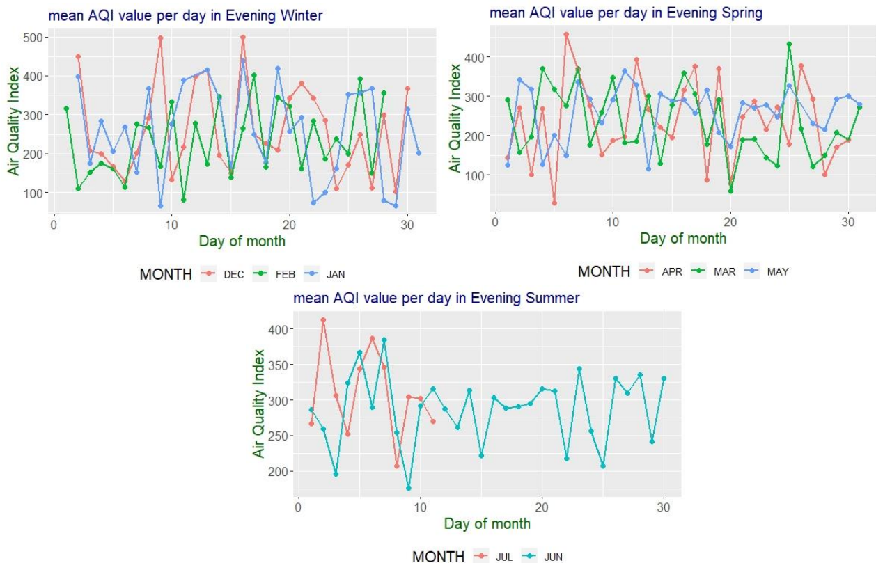
Γράφημα 27: Γραφήματα μέσων τιμών AQI τις απογευματινές ώρες ανά εποχή.
