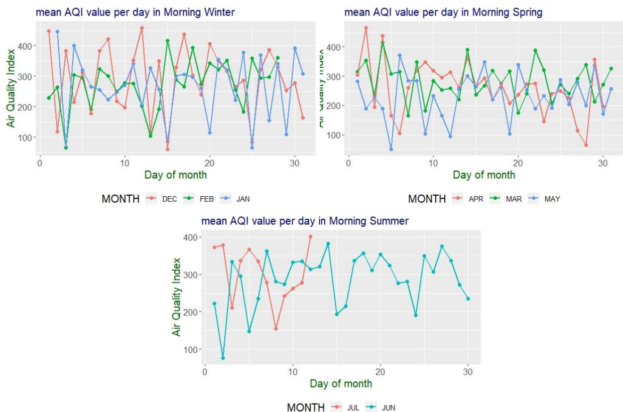
Γράφημα 23: Γραφήματα μέσων τιμών AQI τις πρωινές ώρες ανά εποχή.
